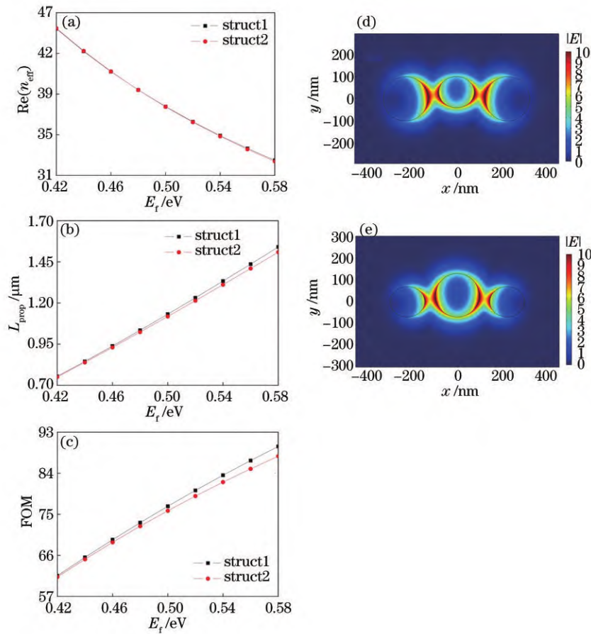
图 11 两种结构所支持的模式 1 的有效折射率实部 Re(n_{eff}) 、传播长度 L_{prop} 和品质因数 FOM 随费米能 E_f 的变化关系对比图, 以及 struct1 和 struct2 所支持的模式 1 在费米能为 0.58 eV 处的电场强度分布图。(a) 有效折射率实部 Re(n_{eff}) ; (b) 传播长度 L_{prop} ; (c) 品质因数 FOM; (d) struct1 和 (e) struct2 所支持的模式 1 在费米能 0.58 eV 处的电场强度分布图
