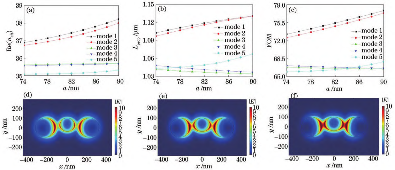
图 6 5 个最低阶模式的有效折射率实部 Re(n_{eff}) 、传播长度 L_{prop} 和品质因数 FOM 随椭圆纳米线半长轴 a 的变化, 以及模式 1 在半长轴为 74 nm、82 nm 和 90 nm 情况下的电场强度分布图。(a) 有效折射率实部 Re(n_{eff}) ; (b) 传播长度 L_{prop} ; (c) 品质因数 FOM; 模式 1 在半长轴 a 为 (d) 74 nm、(e) 82 nm 和 (f) 90 nm 情况下的电场强度分布图
