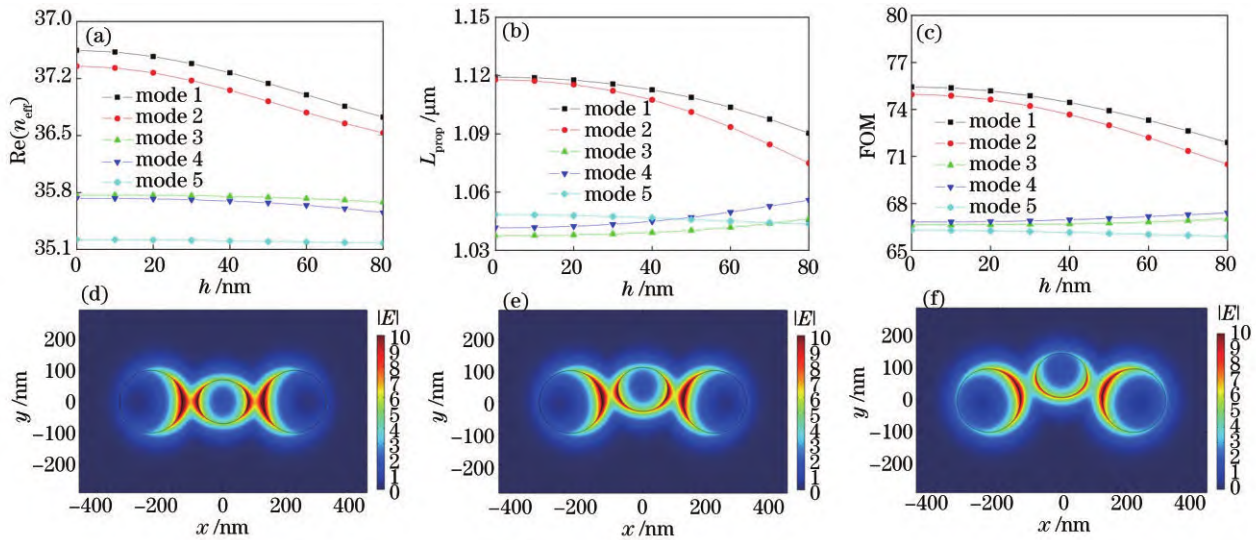
图 9 5 个最低阶模式的有效折射率实部 \text{Re}(n_{\text{eff}}) 、传播长度 L_{\text{prop}} 和品质因数 FOM 随高度 h 的变化, 以及模式 1 在圆柱纳米线高度为 0 nm, 40 nm 和 80 nm 情况下的电场强度分布图。(a) 有效折射率实部 \text{Re}(n_{\text{eff}}) ; (b) 传播长度 L_{\text{prop}} ; (c) 品质因数 FOM; 模式 1 在圆柱纳米线高度 h 为 (d) 0 nm, (e) 40 nm 和 (f) 80 nm 情况下的电场强度分布图
