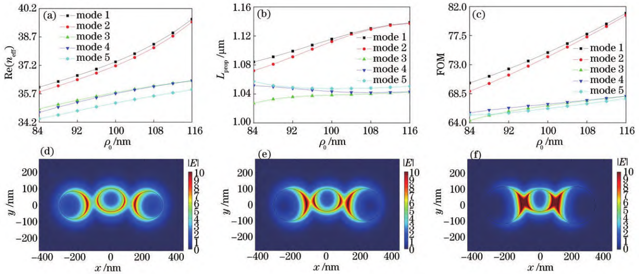
图 5 5 个最低阶模式的有效折射率实部 Re(n_{eff}) 、传播长度 L_{prop} 和品质因数 FOM 随半径 \rho_0 的变化, 以及模式 1 在圆柱半径为 84 nm、100 nm 和 116 nm 时的电场强度分布图。(a)有效折射率实部 Re(n_{eff}) ; (b)传播长度 L_{prop} ; (c)品质因数 FOM; 模式 1 在圆柱半径 \rho_0 为 (d) 84 nm、(e) 100 nm 和 (f) 116 nm 时的电场强度分布图
