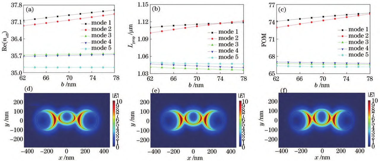
图 7 5 个最低阶模式的有效折射率实部 Re(n_{eff}) 、传播长度 L_{prop} 和品质因数 FOM 随椭圆纳米线半短轴 b 的变化, 以及模式 1 在半短轴 b 为 62 nm、70 nm 和 78 nm 情况下的电场强度分布图。(a) 有效折射率实部 Re(n_{eff}) ; (b) 传播长度 L_{prop} ; (c) 品质因数 FOM; 模式 1 在半短轴 b 为 (d) 62 nm、(e) 70 nm 和 (f) 78 nm 情况下的电场强度分布图
