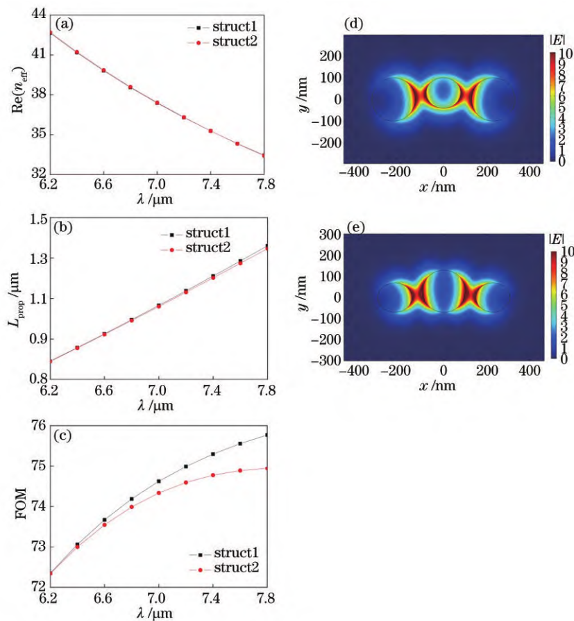
图 10 两种结构所支持的模式 1 的有效折射率实部 \text{Re}(n_{\text{eff}}) 、传播长度 L_{\text{prop}} 和品质因数 FOM 随工作波长 \lambda 的变化关系对比图,以及 struct1 和 struct2 所支持的模式 1 在波长为 7.8 \mu\text{m} 处的电场强度分布图。(a) 有效折射率实部 \text{Re}(n_{\text{eff}}) ; (b) 传播长度 L_{\text{prop}} ; (c) 品质因数 FOM; (d) struct1 和 (e) struct2 所支持的模式 1 在波长为 7.8 \mu\text{m} 处的电场强度分布图
