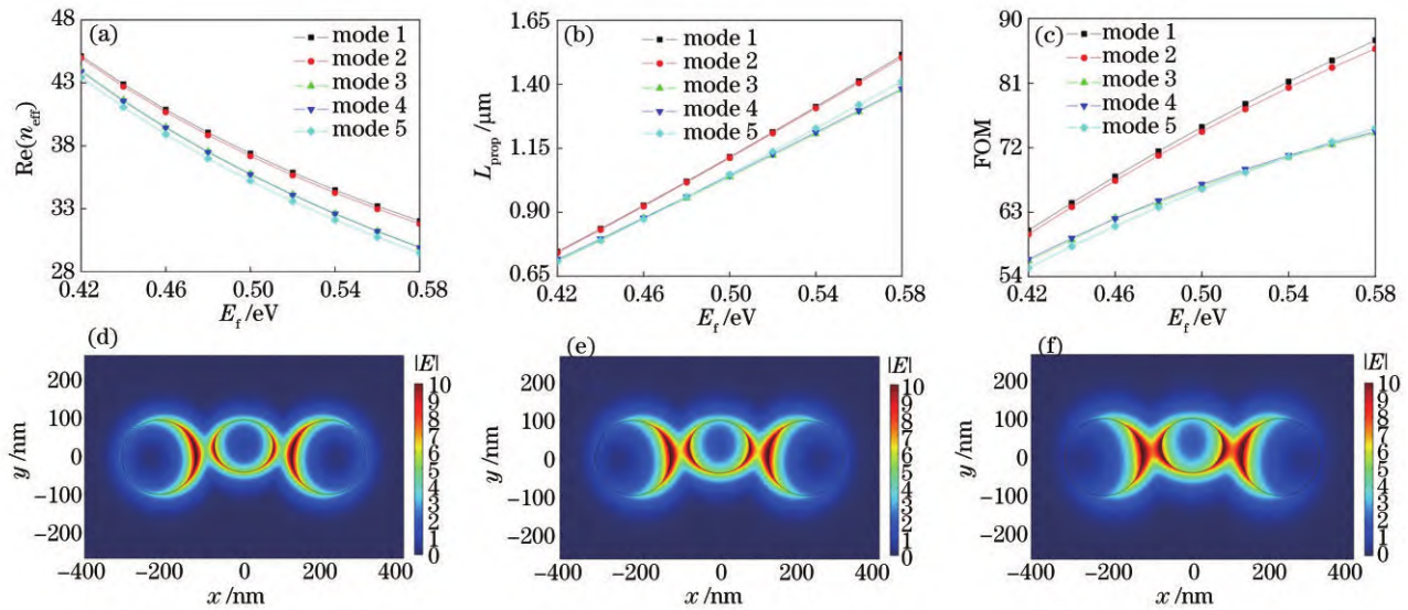
图 4 5 个最低阶模式的有效折射率实部 Re(n_{eff}) 、传播长度 L_{prop} 和品质因数 FOM 随费米能 E_f 的变化, 以及模式 1 在费米能为 0.42 eV、0.50 eV 和 0.58 eV 情况下的电场强度分布图。(a)有效折射率实部 Re(n_{eff}) ; (b)传播长度 L_{prop} ; (c)品质因数 FOM; 模式 1 在费米能 E_f 为 (d) 0.42 eV、(e) 0.50 eV 和 (f) 0.58 eV 情况下的电场强度分布图
